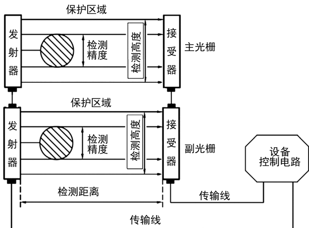
级连式安全光栅工作示意图
