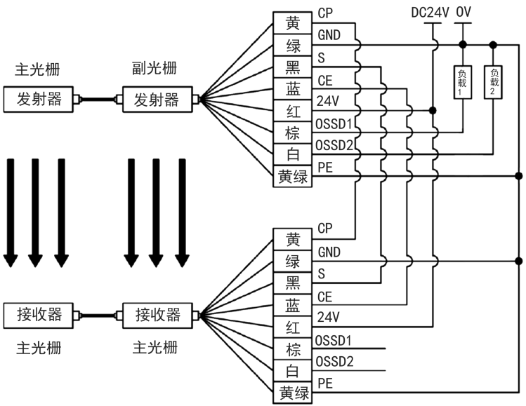
PNP输出型接线图
